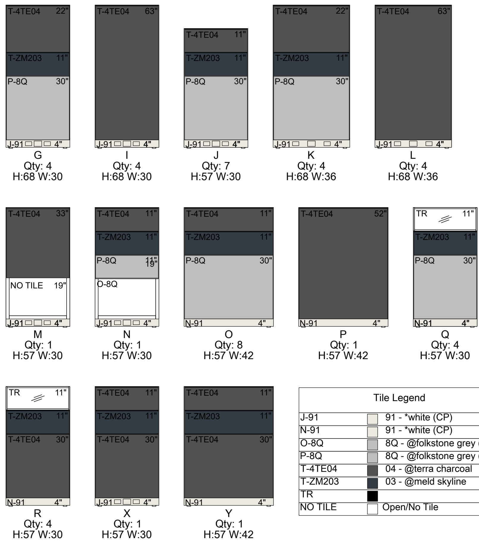
Tile Elevation
